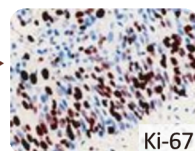
Ki-67
