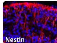
Nestin
